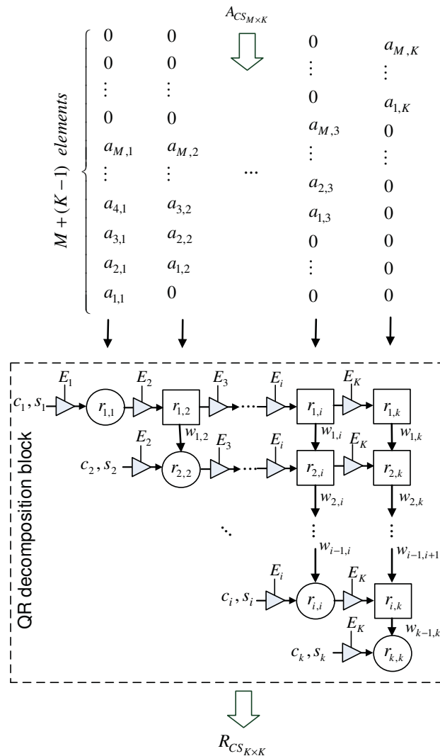
Slika 6.3: Blok za QR dekompoziciju
