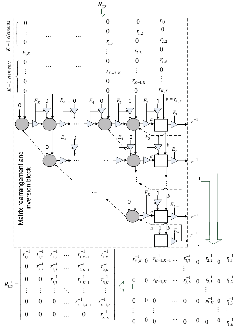
Slika 6.4: Blok za računanje inverzne matrice
