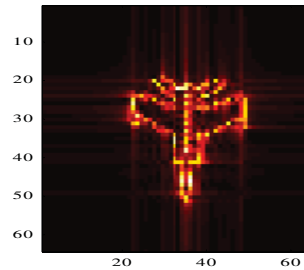
Slika 3.5: ISAR slika Mig25
