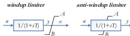
Slika 1.2.9 Osnovni tipovi ograničavača.
