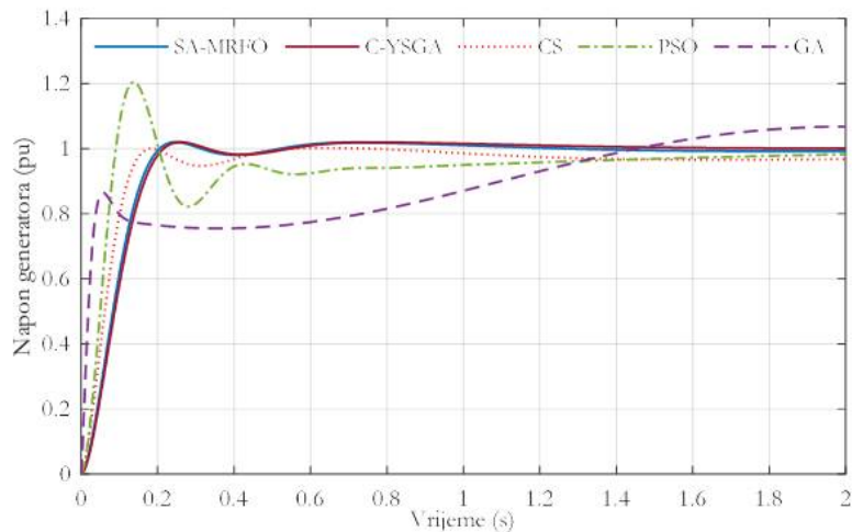
Slika 3.1.10 Poređenje step odziva za različite FOPID regulatore
