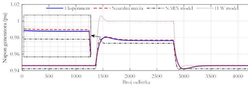
Slika 6.2.8 Poređenje odziva napona generatora – validacioni test 4
