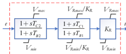
Slika 1.2.12 Blok dijagram lead-lag kompenzatora.
