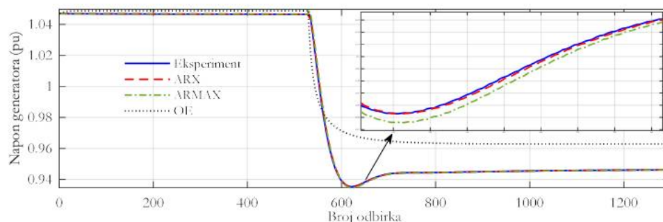
Slika 6.3.4 Poređenje odziva napona generatora – validacioni test 1
