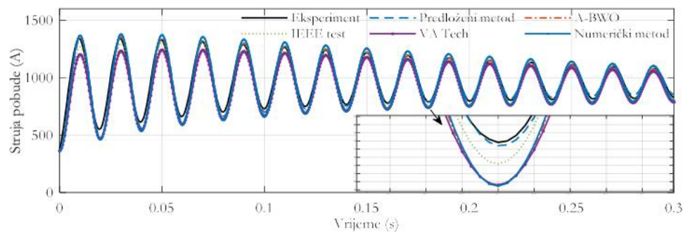
Slika 4.2.20 Grafičko poređenje talasnih oblika struje pobude prilikom oglada kratkog spoja (pri naponu generatora koji iznosi 50% nominalne vrijednosti)
