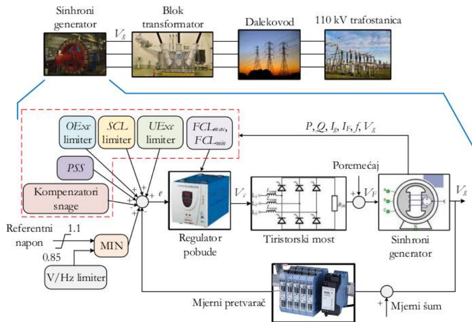
Slika 3.2.1 Blok dijagram simulacionog modela
