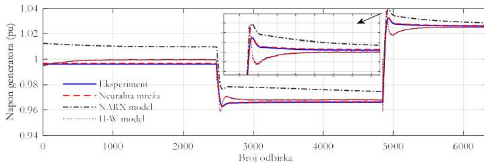
Slika 6.2.6 Poređenje odziva napona generatora – validacioni test 2
