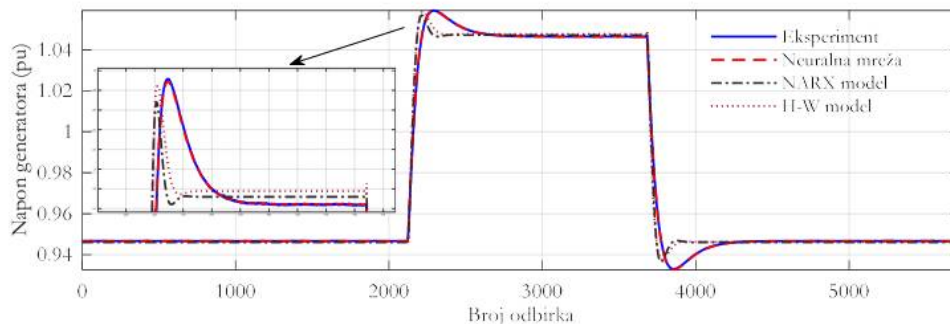
Slika 6.2.5 Poređenje odziva napona generatora – validacioni test 1
