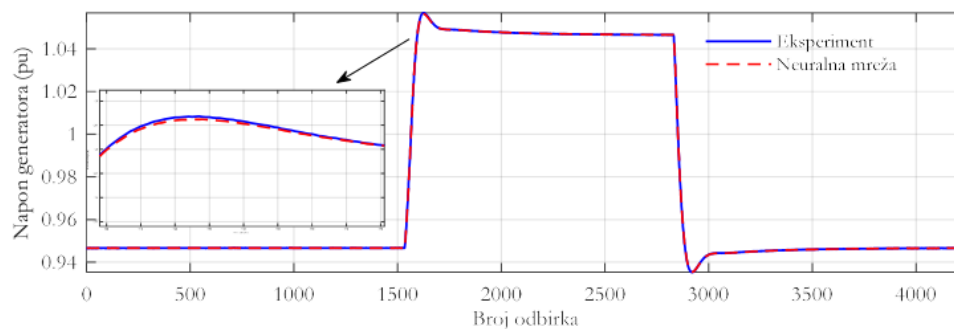
Slika 6.2.4 Grafičko poređenje eksperimentalno snimljenog napona generatora i odgovarajućeg napona dobijenog pomoću obučene neuralne mreže
