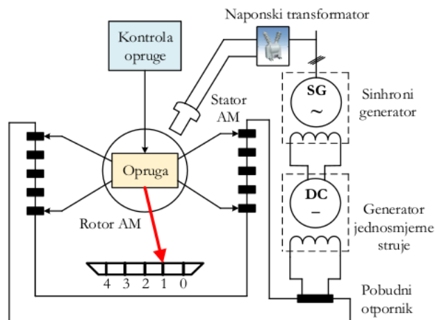
Slika 1.2.3 Principijelna šema brzog sektorskog otpornika.
