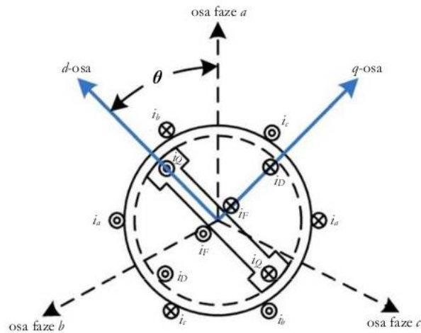
Slika 1.4.2 Ilustracija položaja namotaja i osa sinhronog generatora.
