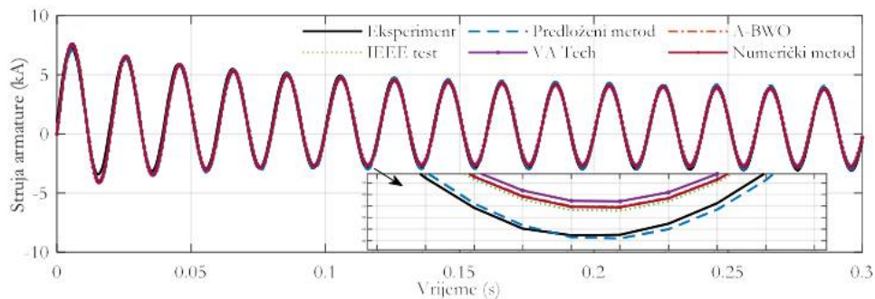
Slika 4.2.6 Grafičko poređenje talasnih oblika struje armature prilikom oglada kratkog spoja (pri naponu generatora koji iznosi 20% nominalne vrijednosti)
