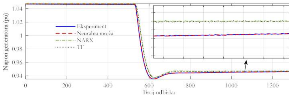
Slika 6.3.8 Poređenje odziva napona generatora – validacioni test 1
