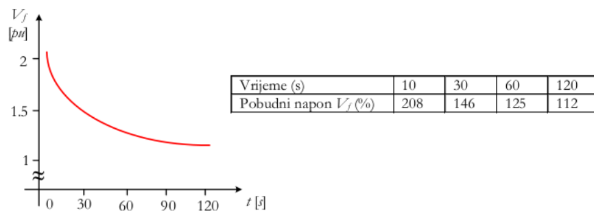
Slika 1.2.14 Tipična kriva maksimalno dozvoljene pobude.
