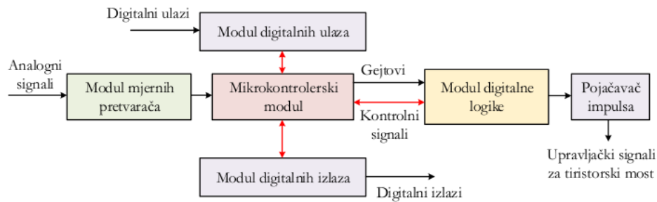
Slika 1.2.6 Blok dijagram mikroprocesorskog regulatora pobude.
