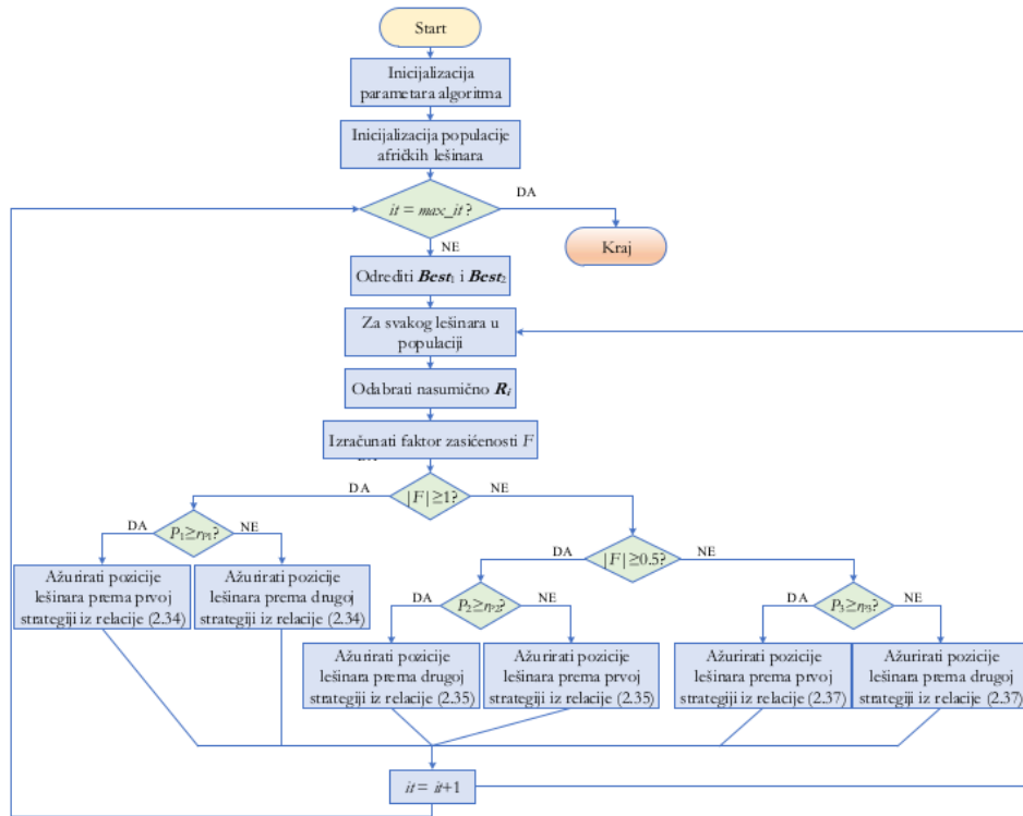
Slika 2.1.14 Dijagram toka algoritma optimizacije pomoću afričkih lešinara
