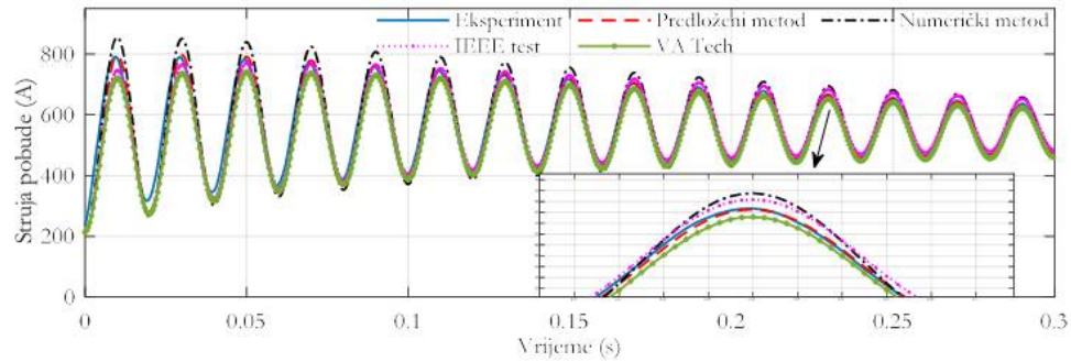
Slika 4.2.2 Grafičko poređenje talasnih oblika pobudne struje prilikom oglada kratkog spoja (pri naponu generatora koji iznosi 30% nominalne vrijednosti)
