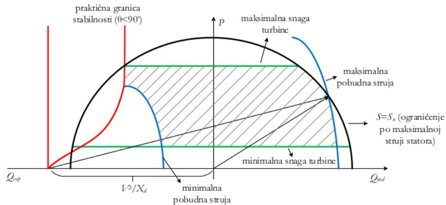
Slika 1.2.13 Pogonski dijagram hidrogenatora.
