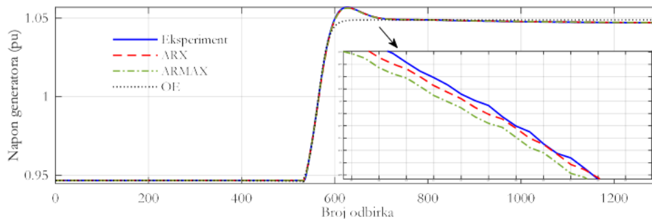
Slika 6.3.3 Grafičko poređenje eksperimentalno snimljenog napona generatora i odgovarajućeg napona dobijenog pomoću obučanih neuralnih mreža
