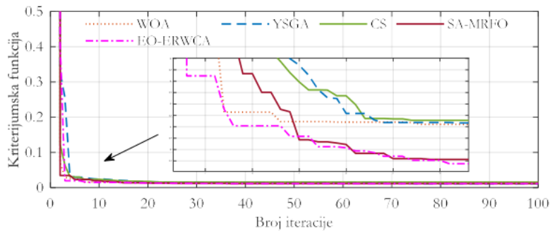
Slika 3.1.25 Poređenje konvergencijskih karakteristika algoritama
