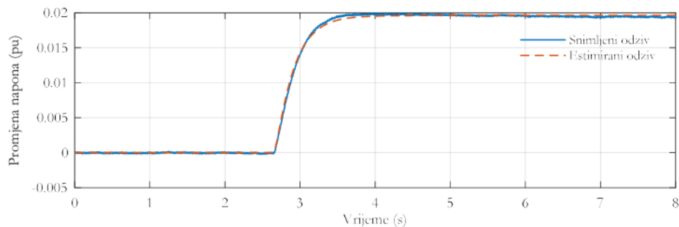
Slika 5.2.9 Grafičko poređenje dobijenih odziva promjene napona generatora
