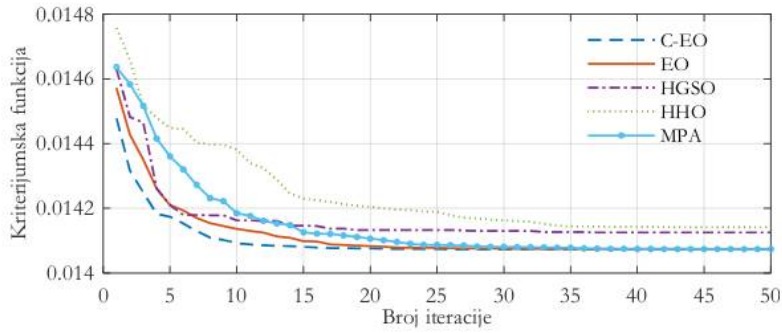
Slika 4.2.8 Konvergenijske krive algoritama prilikom estimacije parametara sinhronog generatora pomoću struje armature – prvi pristup
