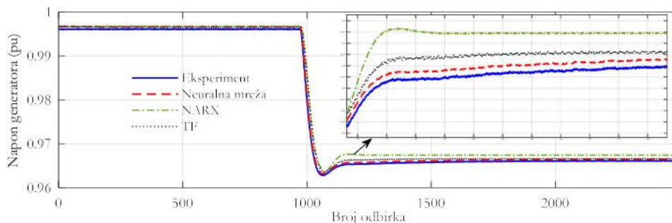
Slika 6.3.9 Poređenje odziva napona generatora – validacioni test 2
