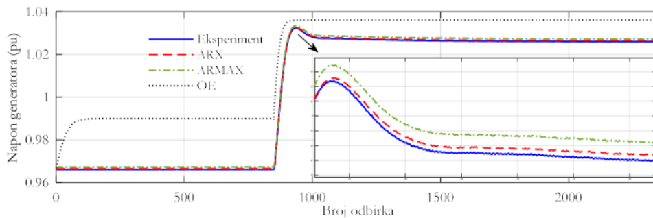
Slika 6.3.6 Poređenje odziva napona generatora – validacioni test 3
