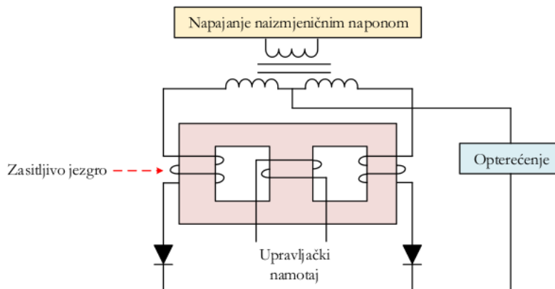
Slika 1.2.4 Struktura magnetnog pojačavača.
