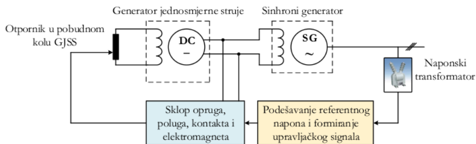
Slika 1.2.1 Principijelna šema Tirill -ovog regulatora.
