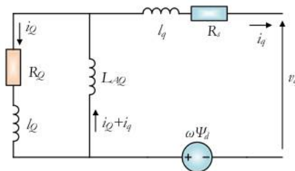
Slika 1.4.4 Ekvivalentno kolo sinhronog generatora po q – osi.
