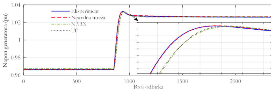
Slika 6.3.10 Poređenje odziva napona generatora – validacioni test 3
