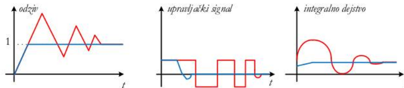
Slika 1.2.10 Ilustracija efekta zasićenja regulatora.
