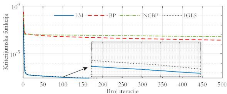
Slika 6.2.3 Konvergencijske krive algoritama za obučavanje neuralne mreže
