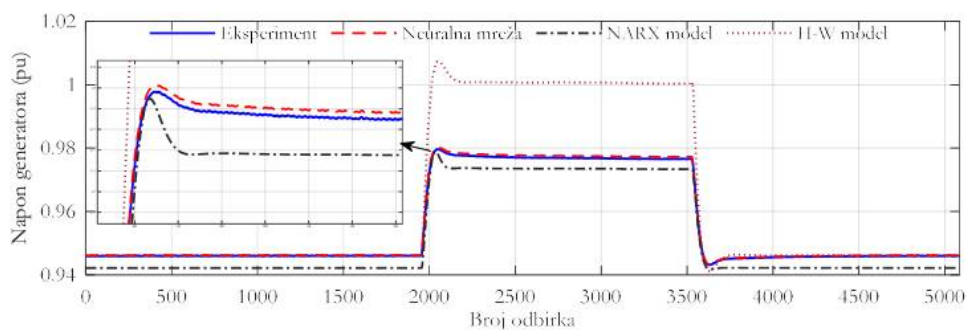
Slika 6.2.7 Poređenje odziva napona generatora – validacioni test 3
