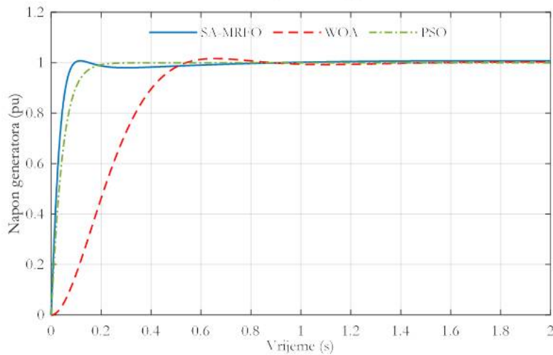
Slika 3.1.15 Poređenje step odziva za različite PIDD 2 regulatore
