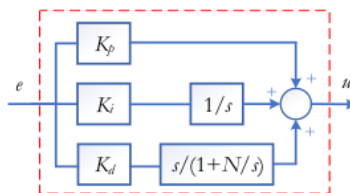
Slika 1.2.8 Blok dijagram realnog PID regulatora.
