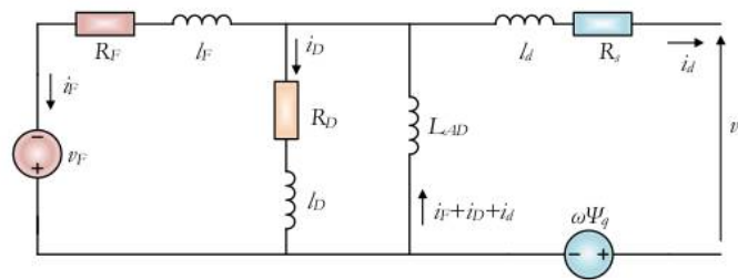
Slika 1.4.3 Ekvivalentno kolo sinhronog generatora po d – osi.
