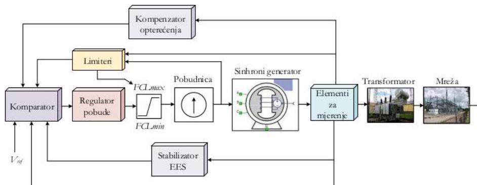
Slika 1.1.2 Detaljan prikaz strukture sistema za regulaciju pobude
