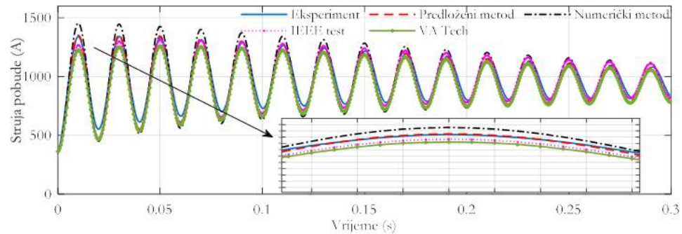
Slika 4.2.3 Grafičko poređenje talasnih oblika pobudne struje prilikom oglada kratkog spoja (pri naponu generatora koji iznosi 50% nominalne vrijednosti)
