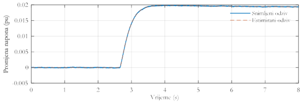
Slika 5.2.8 Grafičko poređenje dobijenih odziva promjene napona generatora
