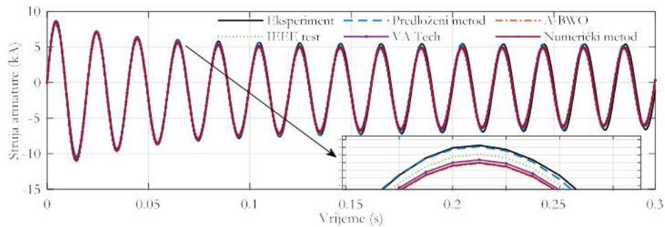
Slika 4.2.5 Grafičko poređenje talasnih oblika struje armature prilikom oglada kratkog spoja (pri naponu generatora koji iznosi 50% nominalne vrijednosti)
