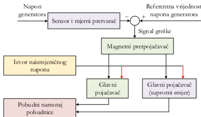
Slika 1.2.5 Blok dijagram regulatora na principu magnetnih pojačavača.
