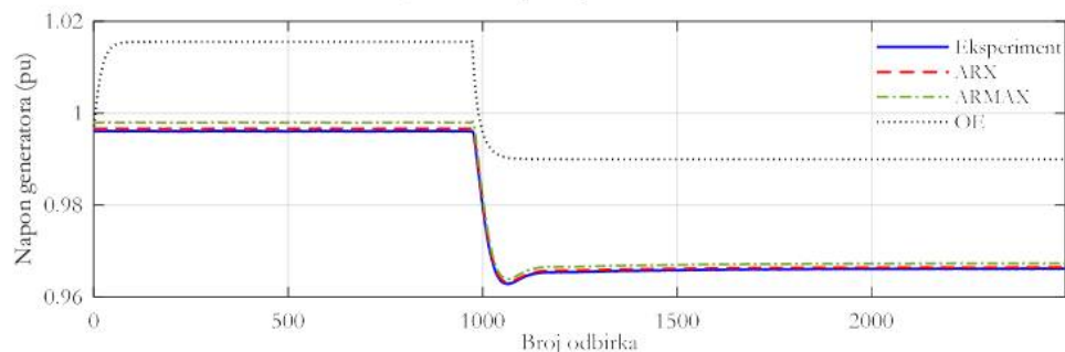
Slika 6.3.5 Poređenje odziva napona generatora – validacioni test 2
