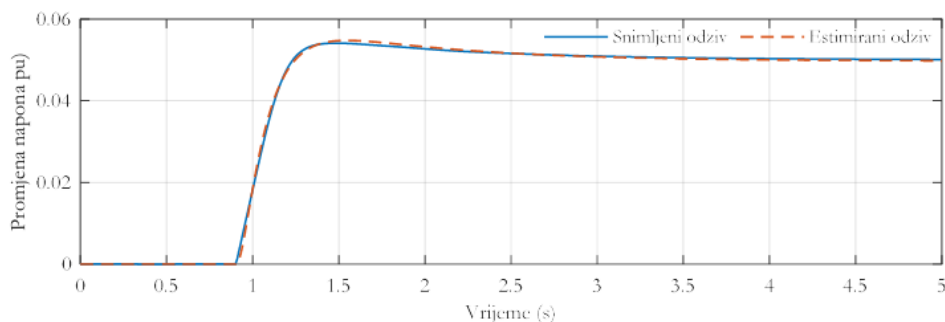
Slika 5.1.5 Grafičko poređenje dobijenih odziva promjene napona generatora
