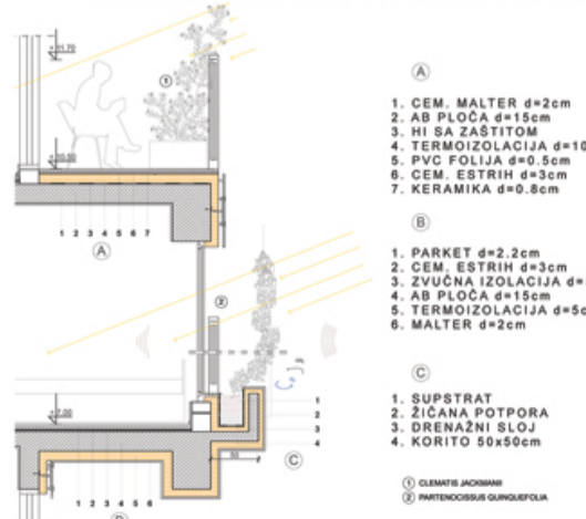
21. Decembar DETALJ OZELENJAVANJA ISTOČNE FASADE
