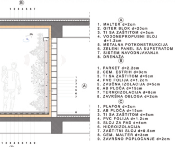
21. Jun DETALJ ZELENOG ZIDA U ZAJEDNIČKOM PROSTORU
