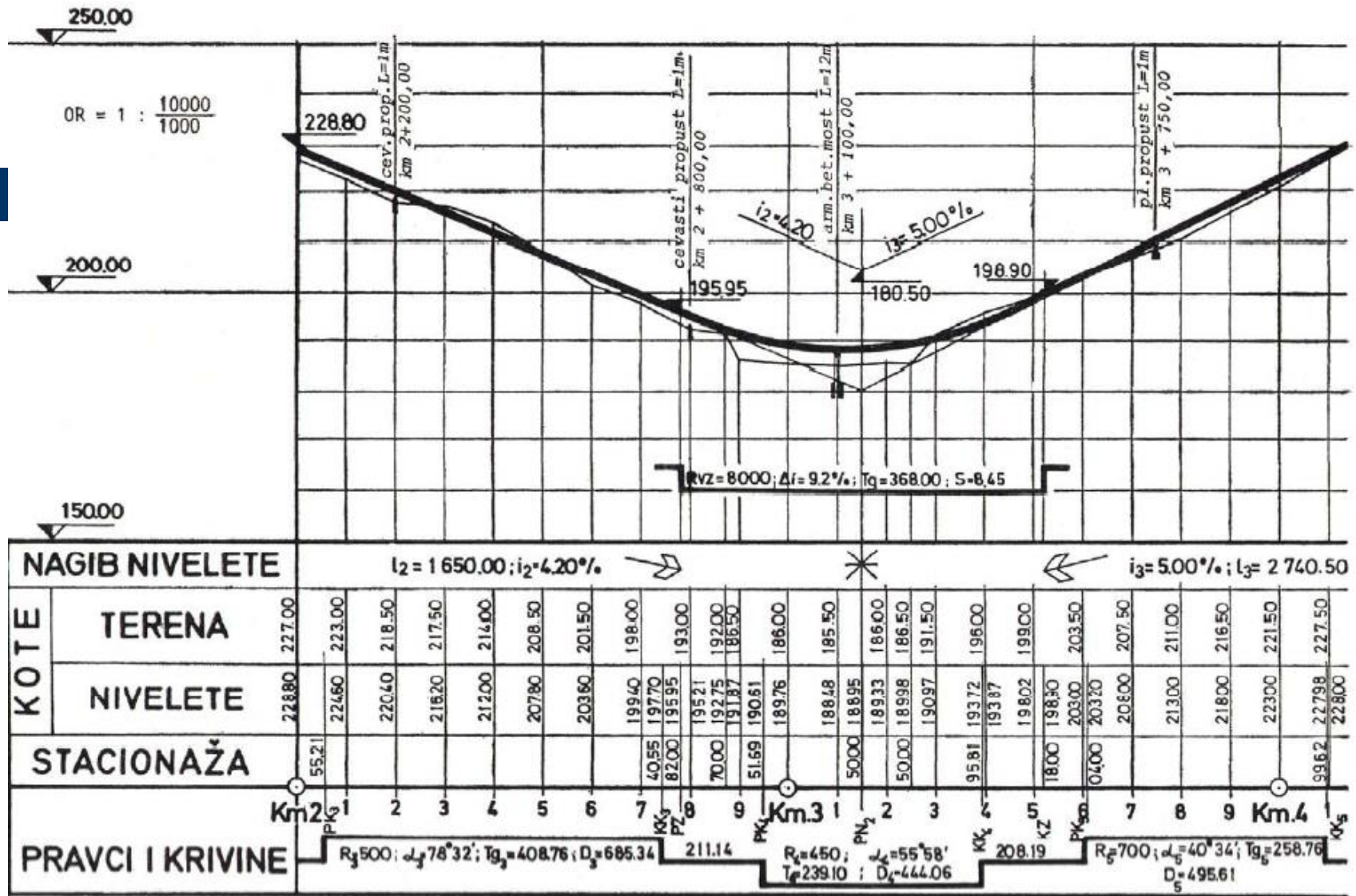
Podužni profil
