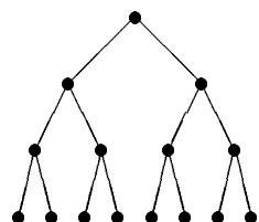
potpuno binarno drvo visine 3
