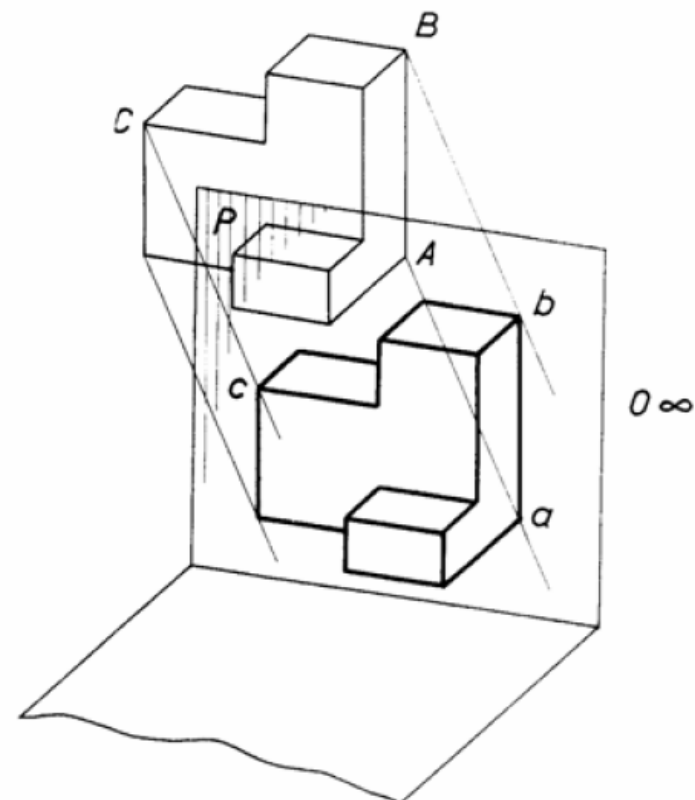
Koso projiciranje
