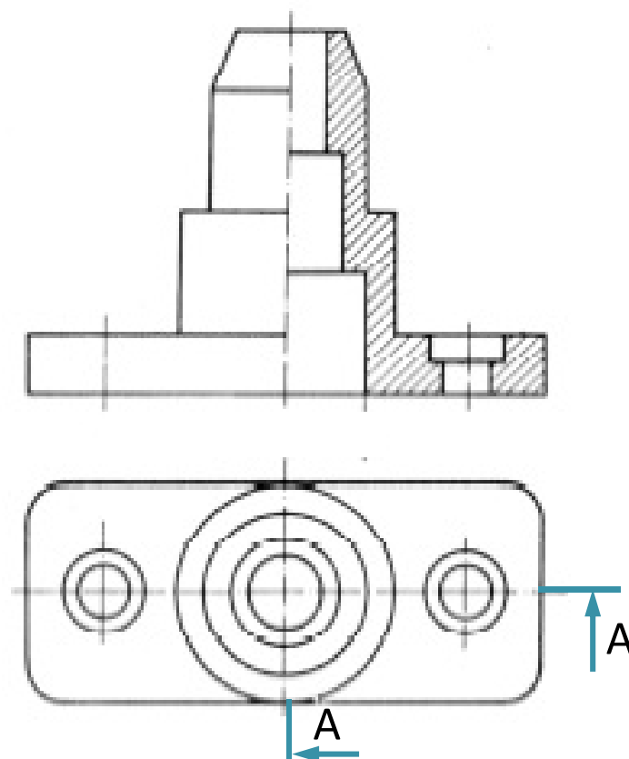
Presjek A-A
