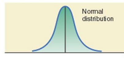
(d) Sampling distribution of \bar{x} for n = 30 .
