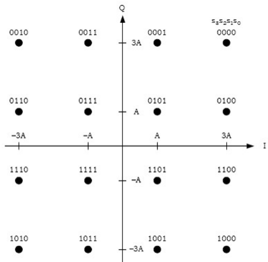
16-QAM (kvadraturna konstelacija)
