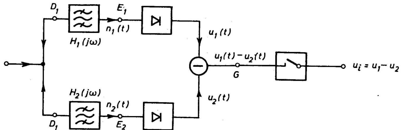
FSK demodulator sa detektorom anvelope – nekoherentni FSK demodulator
