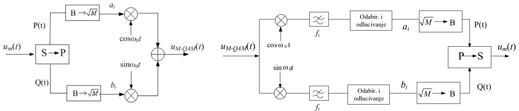
Principska šema predajnika i prijemnika M-QAM signala
