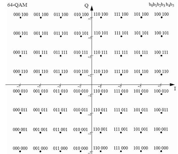
64-QAM
