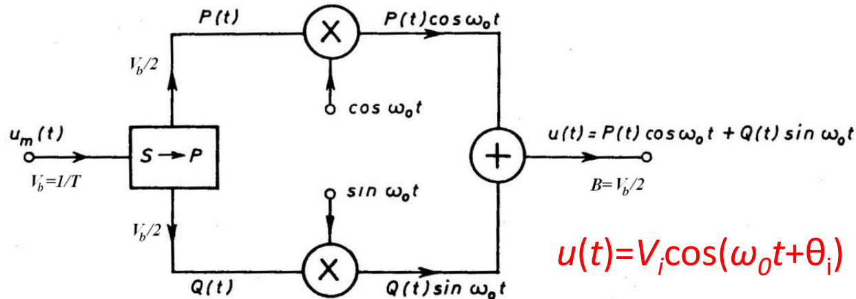
QPSK predajnik
