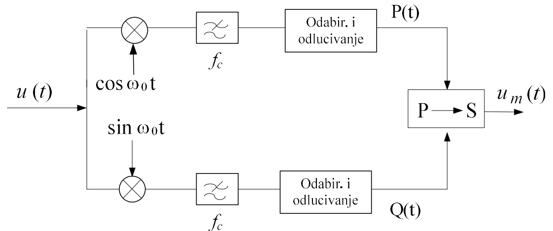
QPSK prijemnik
