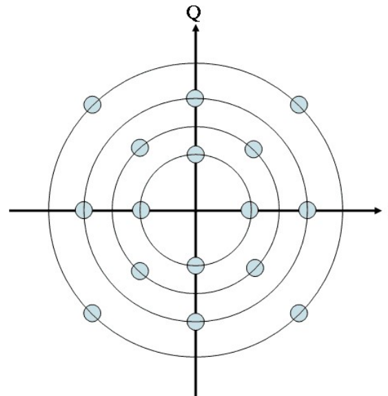
16-QAM (kružna konstelacija)
