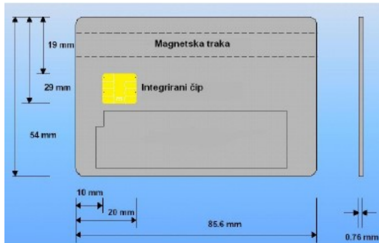
Slika 4.1.1 Standardne dimenzije pametne kartice
