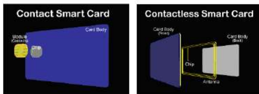
Slika 1.5 Kontaktne i bekontaktne (RF) kartice
