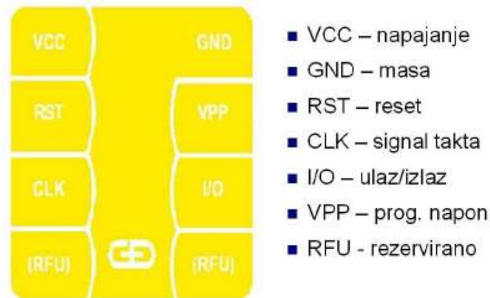
Slika 4.2.3 Izgled i značenje pojedinog kontakta
