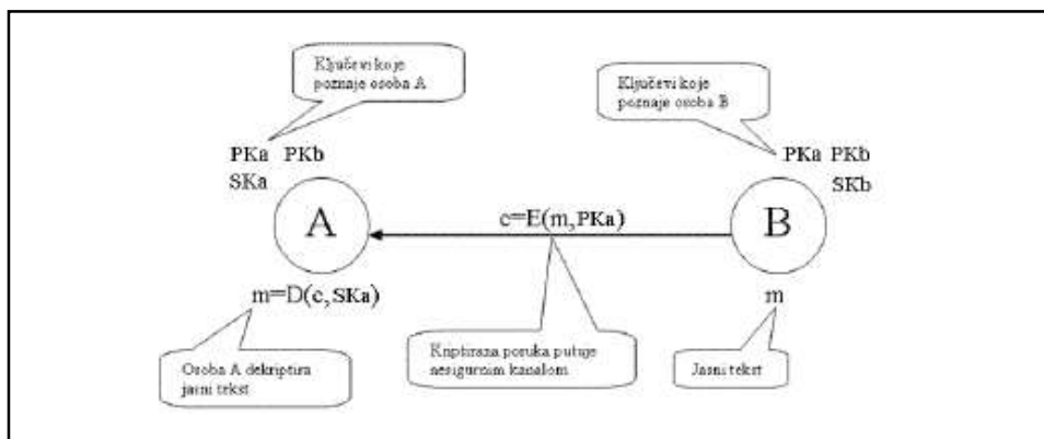
Slika 4.3.21 Šema rada asimetričnog kriptografskog sistema.
