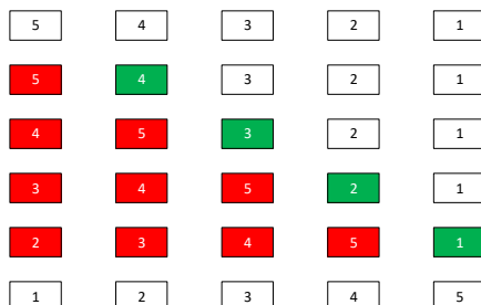
Slika 1: Zelenom bojom označen je tekući element ( array[i] ) dok su crvenom bojom označeni elementi u intervalu 0..i-1 koji su veći od tekućeg odnosno oni koje je za jednu poziciju potrebno pomjeriti udesno.
