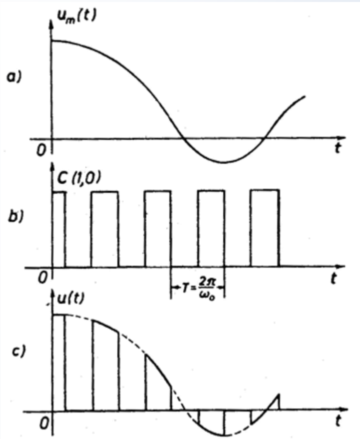
Slika: a) Modulišući signal, b) prekidačka funkcija, c) modulisani signal
