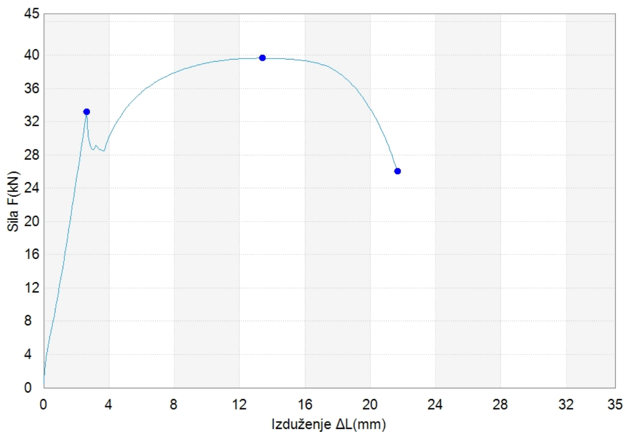
Dijagram istezanja
