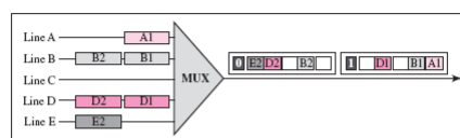
a. Synchronous TDM
